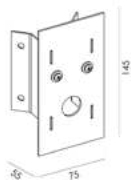
Art. 155 Pièce d'angle pour applique Lofoten sur bras Art. 1939 Art. 1949 Art. 1963 Art. 1969
