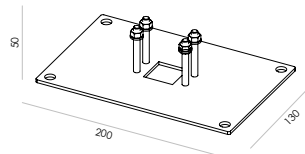
Art. 3081 Semelle pour bornes utilisant normalement 1907ZZ Asker Molde Trysil
