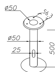
Art. 205ZZ Kit d'ancrage pour béton Alta - Astrid Egersund Mini & Park Halmstad Kisa - Lillesand Lofoten Oppland Stockholm
